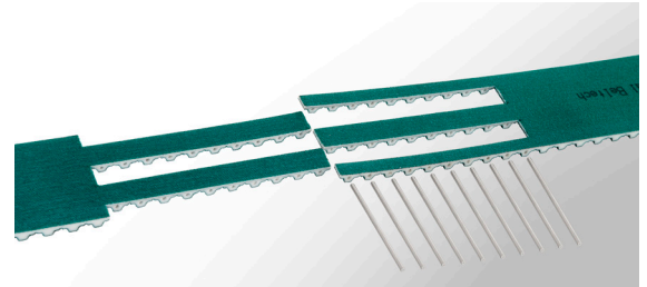
Las correas dentadas con uniones de pasadores vienen con los extremos precortados
