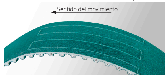
La superficie resultante de la banda es lisa y sin vacíos
