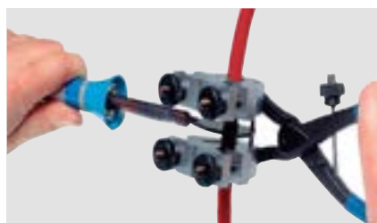
Ręczna zgrzewarka
